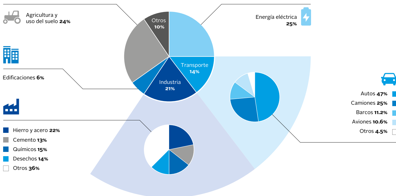
Gráfico 2: Emisiones globales por sector, fuente: Aceleración de la transición al enfoque bajo en carbono de la Institución Brookings
