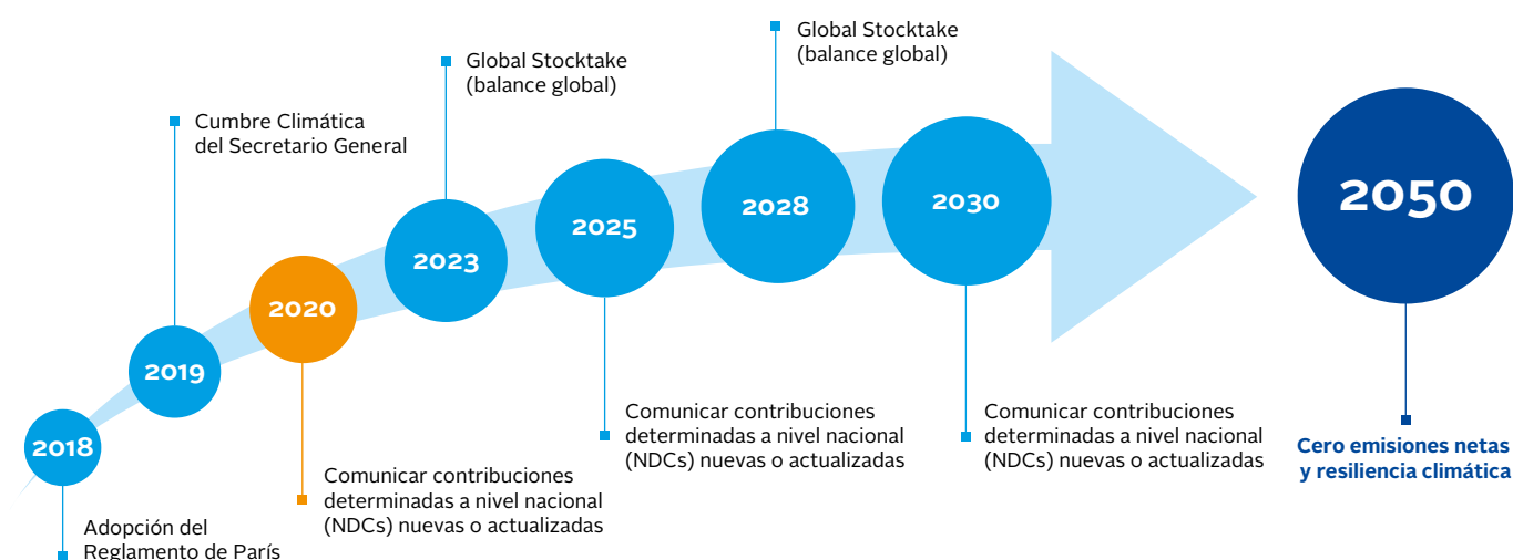
Gráfico 3: Mecanismo de las ambiciones del Acuerdo de París
