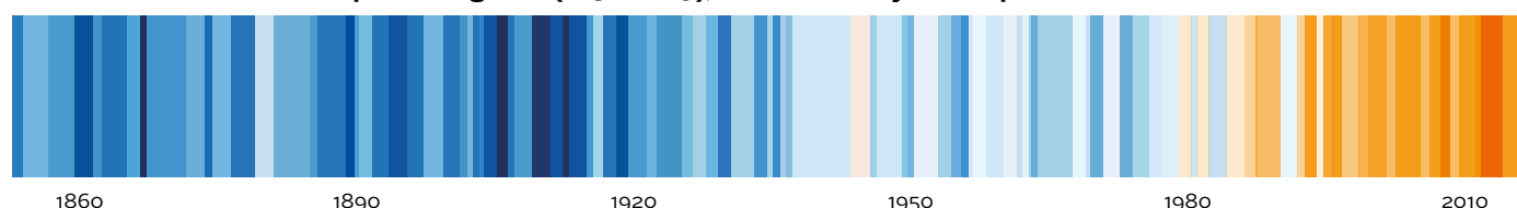
Gráfico 1: Cambio de la temperatura global (1850-2019), fuente: Show your stripes
